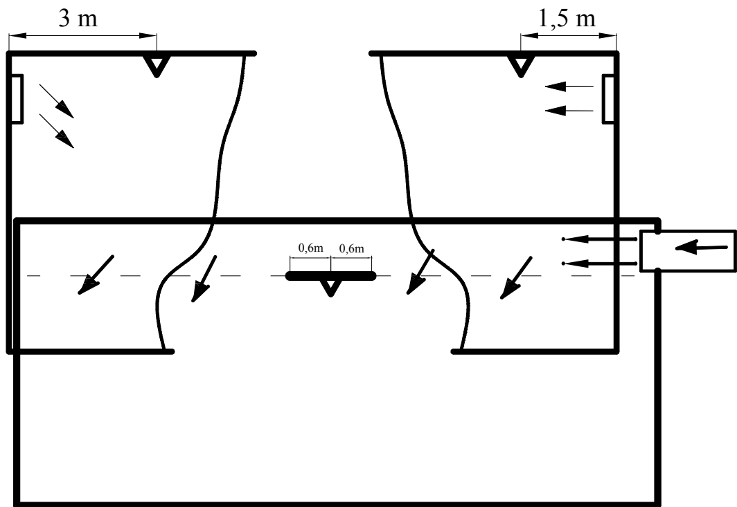
a) vedere în secțiune
