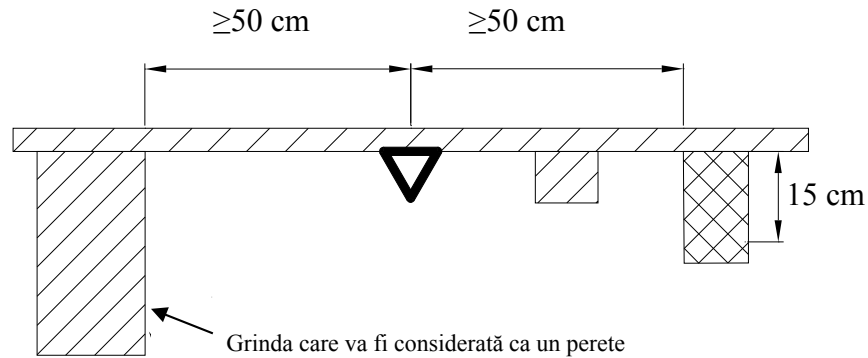
Figura 3.4 Amplasarea detectorului față de elemente de construcții
