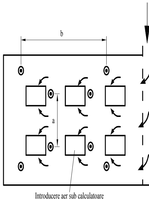
Figura 3.16 Amplasarea detectoarelor în podea falsă, a-distanțe mici și b-distanțe mari
