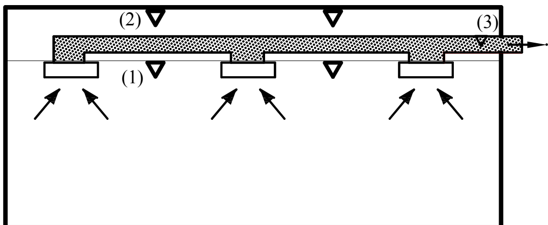
Figura 3.12 Detectoare amplasate simetric între gurile de aspirație montate la nivelul tavanului
