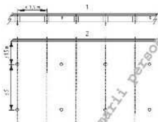
Figura 7.6 Amplasarea sprinklerelor pe traveele drepte formate între grinzile așezate pe o singură direcție, la distanțe sub 1,5 m : 1 – tavan ; 2 – perete
