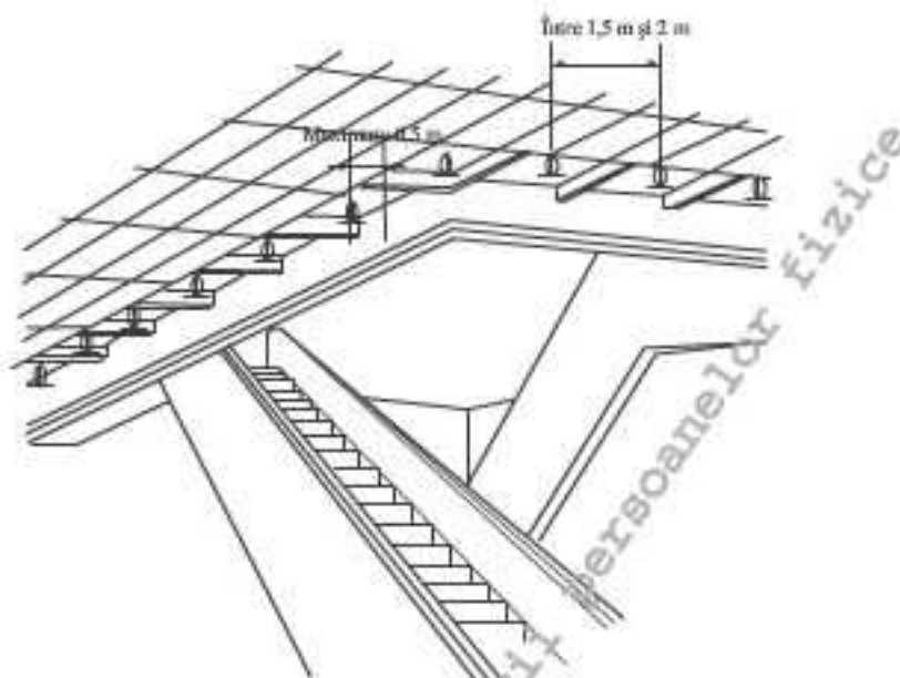
Figura 7.10 Amplasarea sprinklerelor în jurul golurilor din tavane
