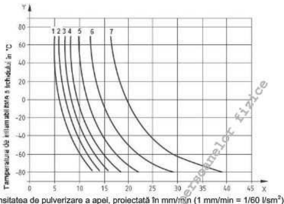
Figura. 8.1 Densitatea de pulverizare a apei pentru stingerea incendiilor de produse petroliere vărsate, pe baza punctelor de inflamabilitate a lichidului.
