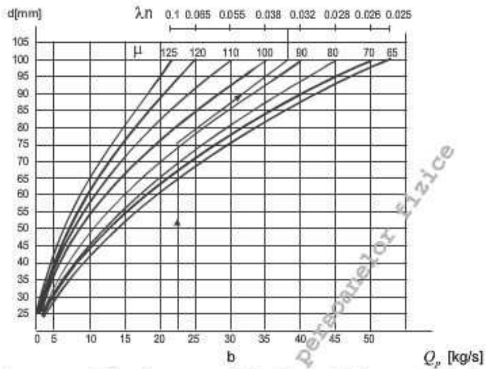
Figura 26.1. Nomograme de dimensionare a conductelor principale de transport a pulberii: a - pentru \lambda_n = 0,0166 \dots 0,063 ; b - pentru \lambda_n = 0,025 \dots 1
