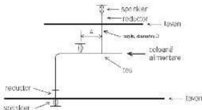
Figura 7.4. Amplasarea sprinklerelor în spațiul dintre nivelul tavanului și al acoperișurilor
